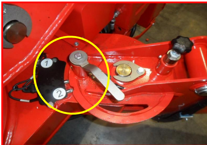
Afbeelding 46: pen stempelpoten.
