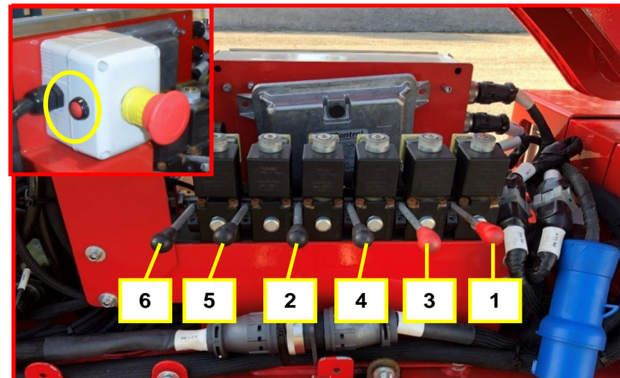
Afbeelding 47: hendels van de hydraulische verdeler.
